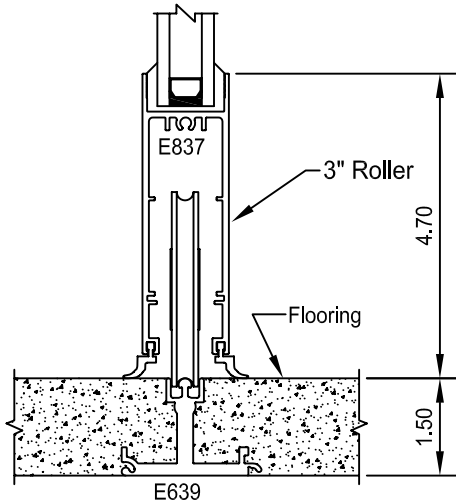
E1 Thin Line Sill Optional 3" Monster Roller
