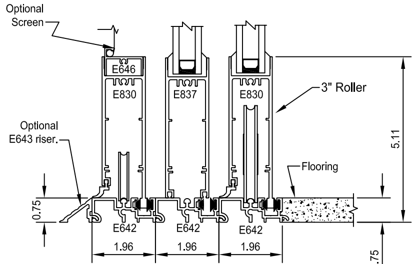
E2 Flush Sill
