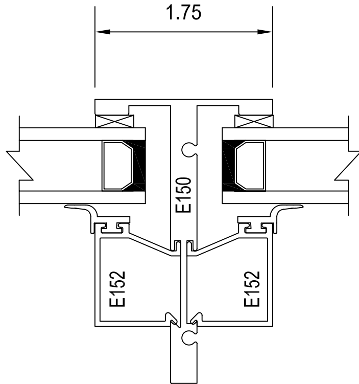
C T-Bar
